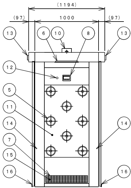
A-A断面
